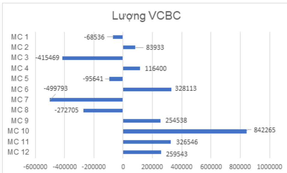
Hình 12: Biểu đồ phân bố lượng vận chuyển bùn cát qua 12 mặt cắt (m 3 /năm).
