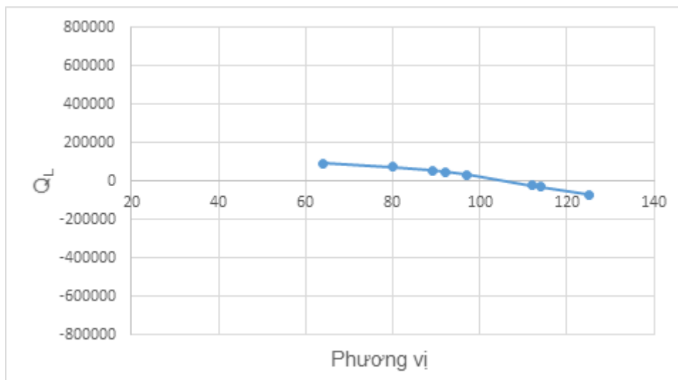
Hình 14: Quan hệ giữa vận chuyển bùn cát và phương vị đường bờ.
