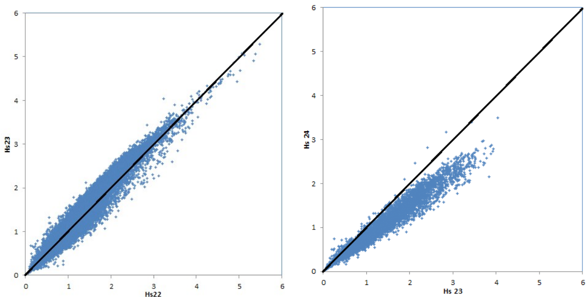
Hình 6. Biểu đồ tương quan chiều cao sóng 22 - 23 và 23 - 24
