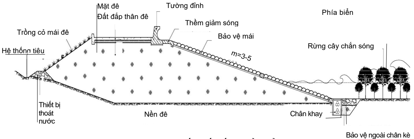
Hình 12 - Mặt cắt thiết kế đê biển điển hình
