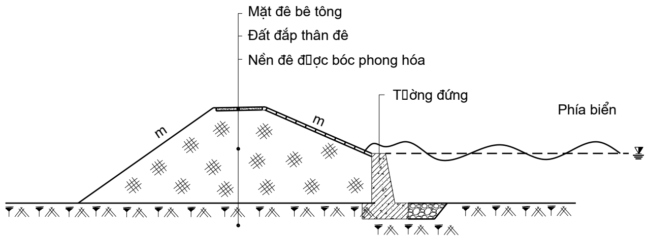
Hình 6 - Mặt cắt ngang đê biển dạng mái nghiêng kết hợp tường đứng
