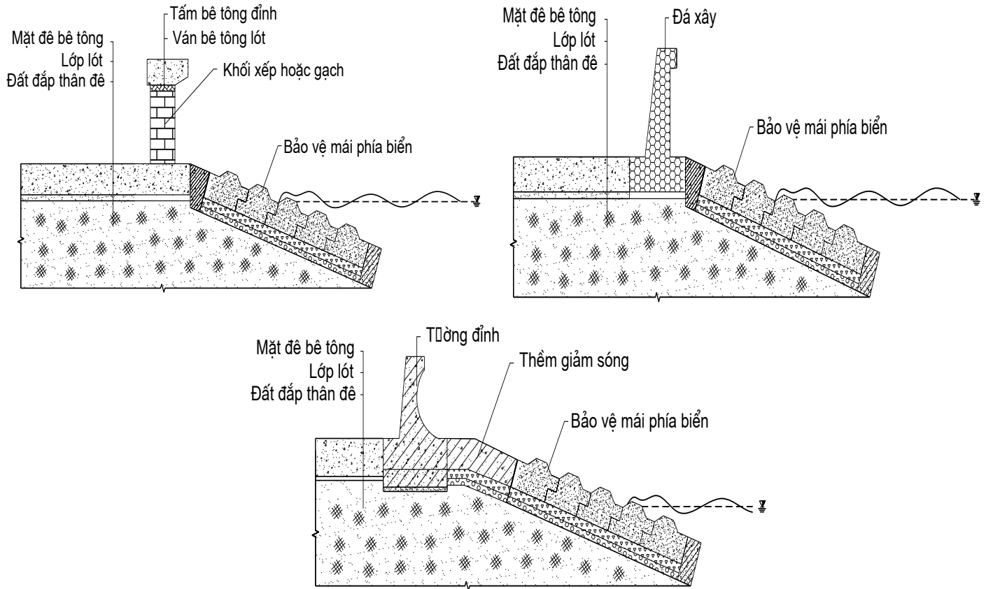
Hình 14 - Một số dạng điển hình về kết cấu tường đỉnh của đê biển
